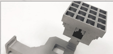
Antena con geometría interna compleja optimizada para fabricación aditiva metálica
